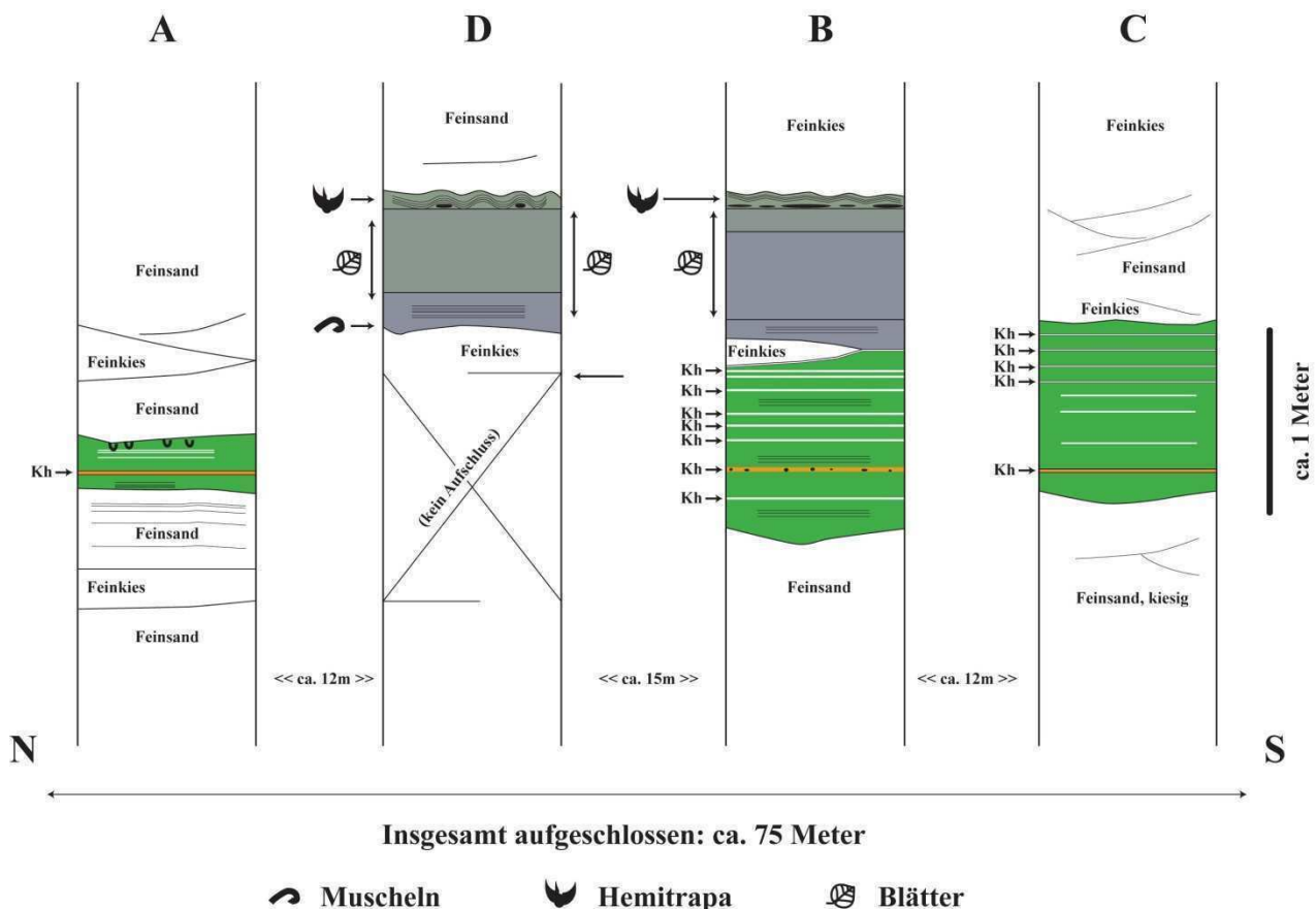
Abb. 2: Skizze der östliche Abbauwand der Kiesgrube Stowasser in Entrischenbrunn mit Einzelprofilen A-D (Kh=kalkige Horizonte)
