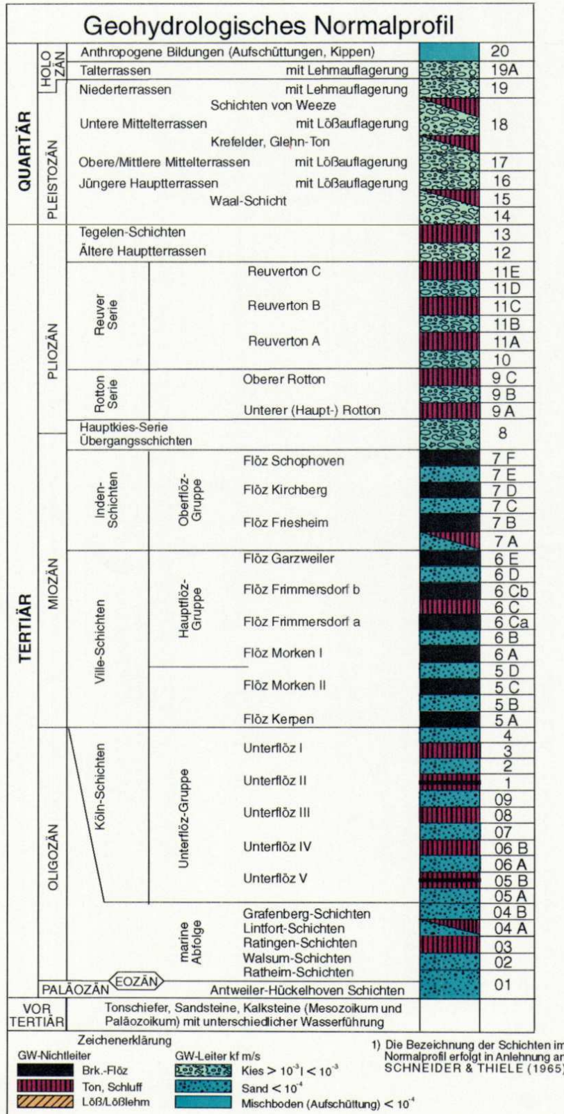
Abb. 2a: Normalprofil Rheinisches Revier,
