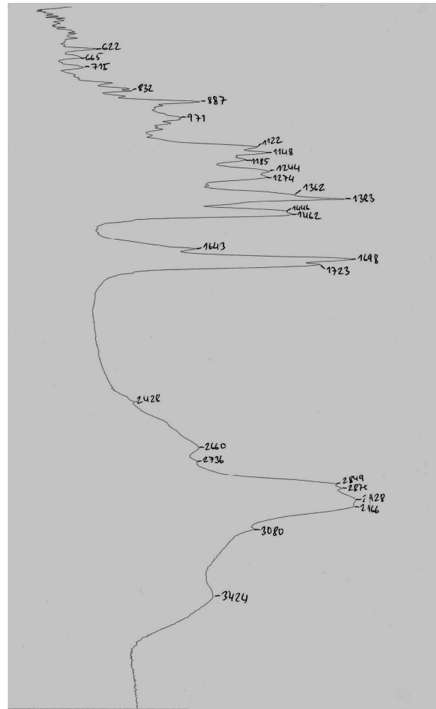
Abb. 2: IR-Spektrum (Wellenzahl der einzelnen Absorptionsmaxima in \text{cm}^{-1} )
