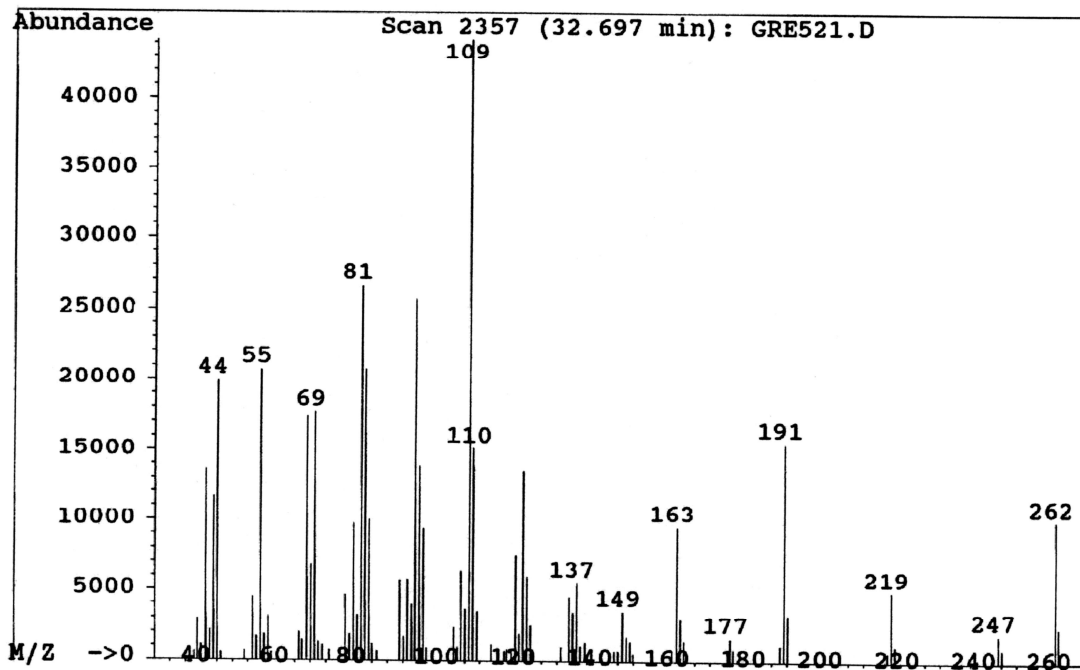
Abb. 4: Nachweis von Norabietan (Ausschnitt des Gesamtionenchromatogramms sowie Massenspektrum).
