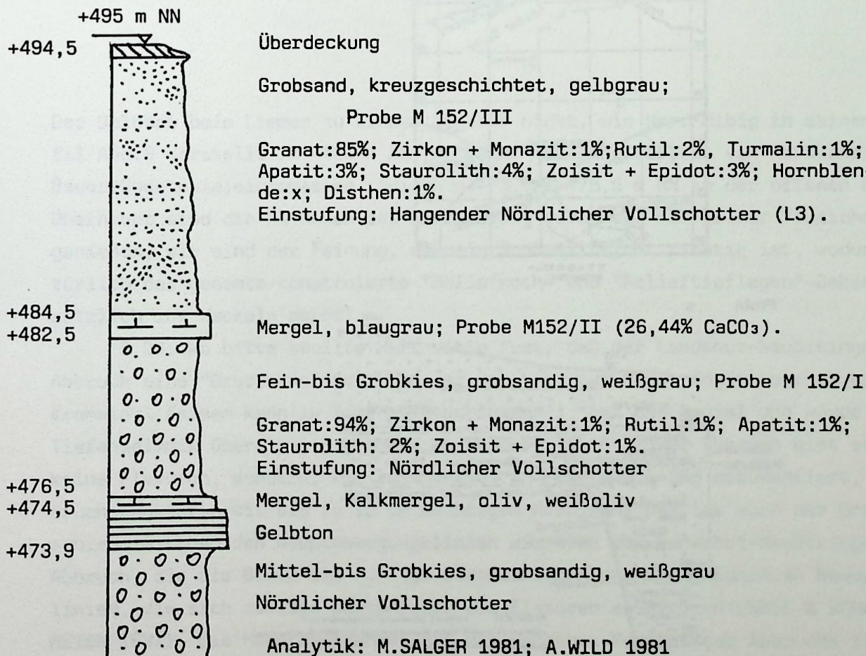
Abb.1. Die Bentonitgrube Limmer zu Linden (Molassebehebung M 152). Profil.
