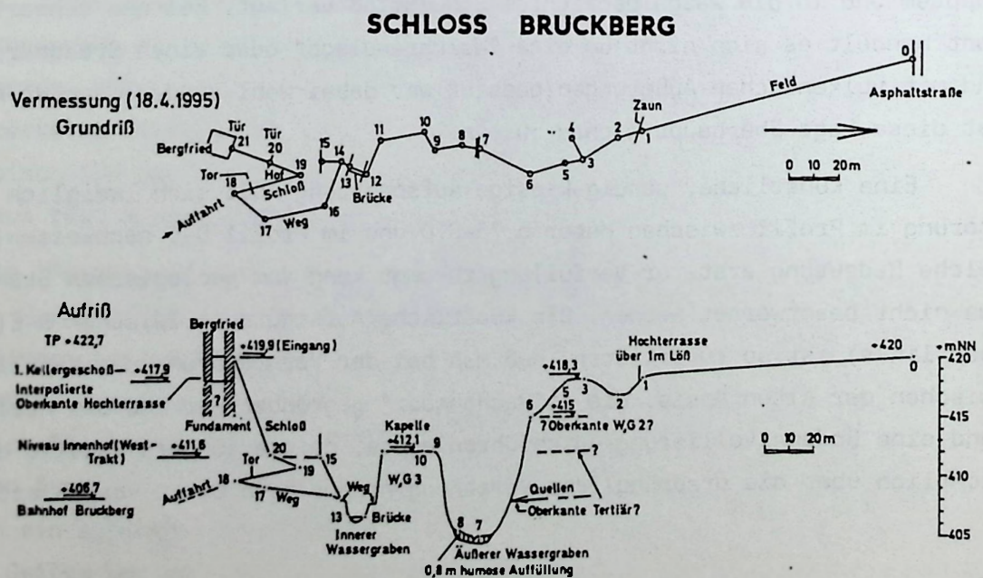
Abb.6. Vermessung und Profil von der Hochterrasse im Norden über die Verebnungen von Schloßkapelle und Schloß bis zum Bergfried
