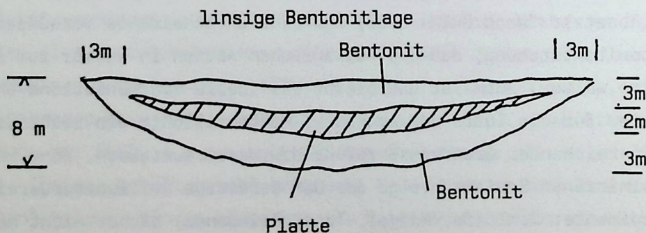
Abb.11. Schematische Darstellung einer linsigen Bentonitlage mit Plattenton im Kern nach der Montmorillonitisierung der Tuffe und Aschen
