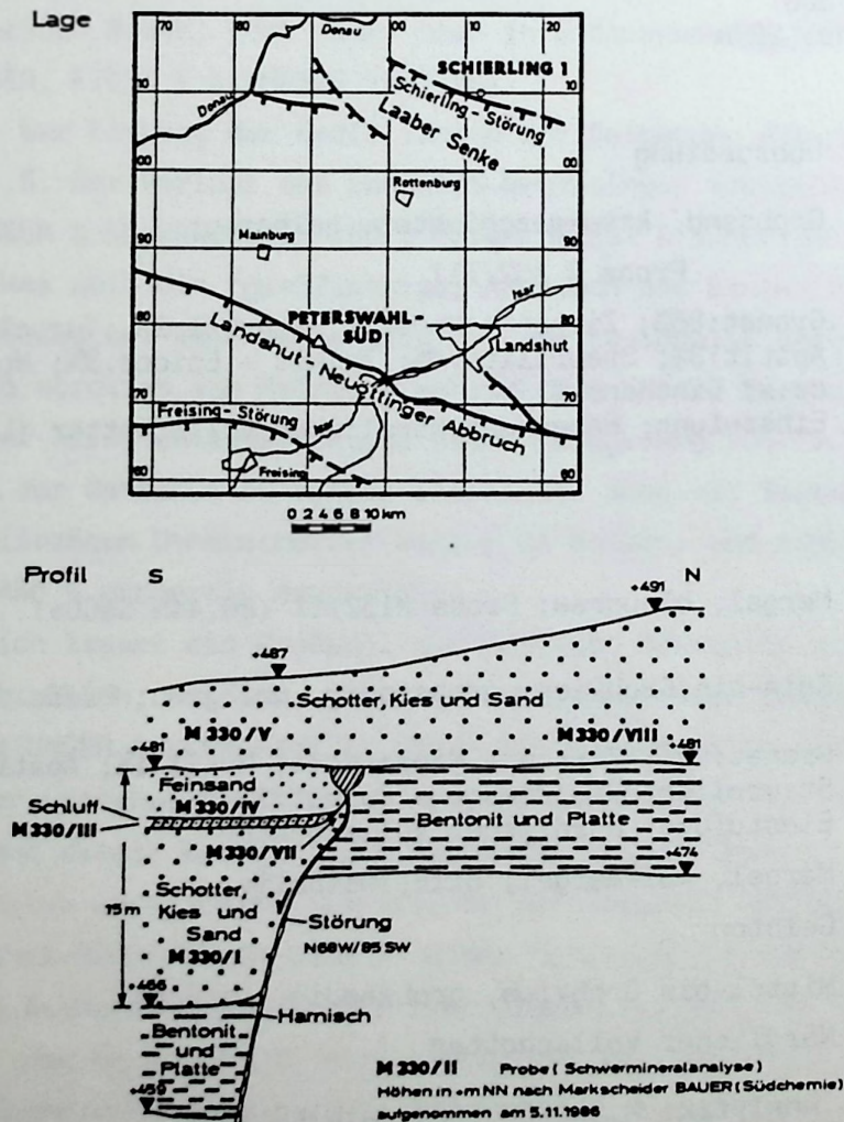
Abb.2. Lage und Profil der Bentonitgrube Peterswahl-Süd (aus: UNGER & SCHWARZMEIER 1987:13).
