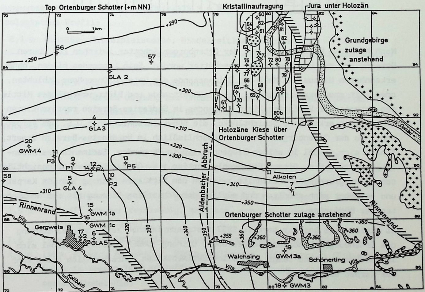
Abb.2. Lage der von der Rhein-Main-Donau A.G. abgeteufte Flachbohrungen (Nr.60 bis 82; am nördlichen Rand der Karte) östlich von Osterhofen.
