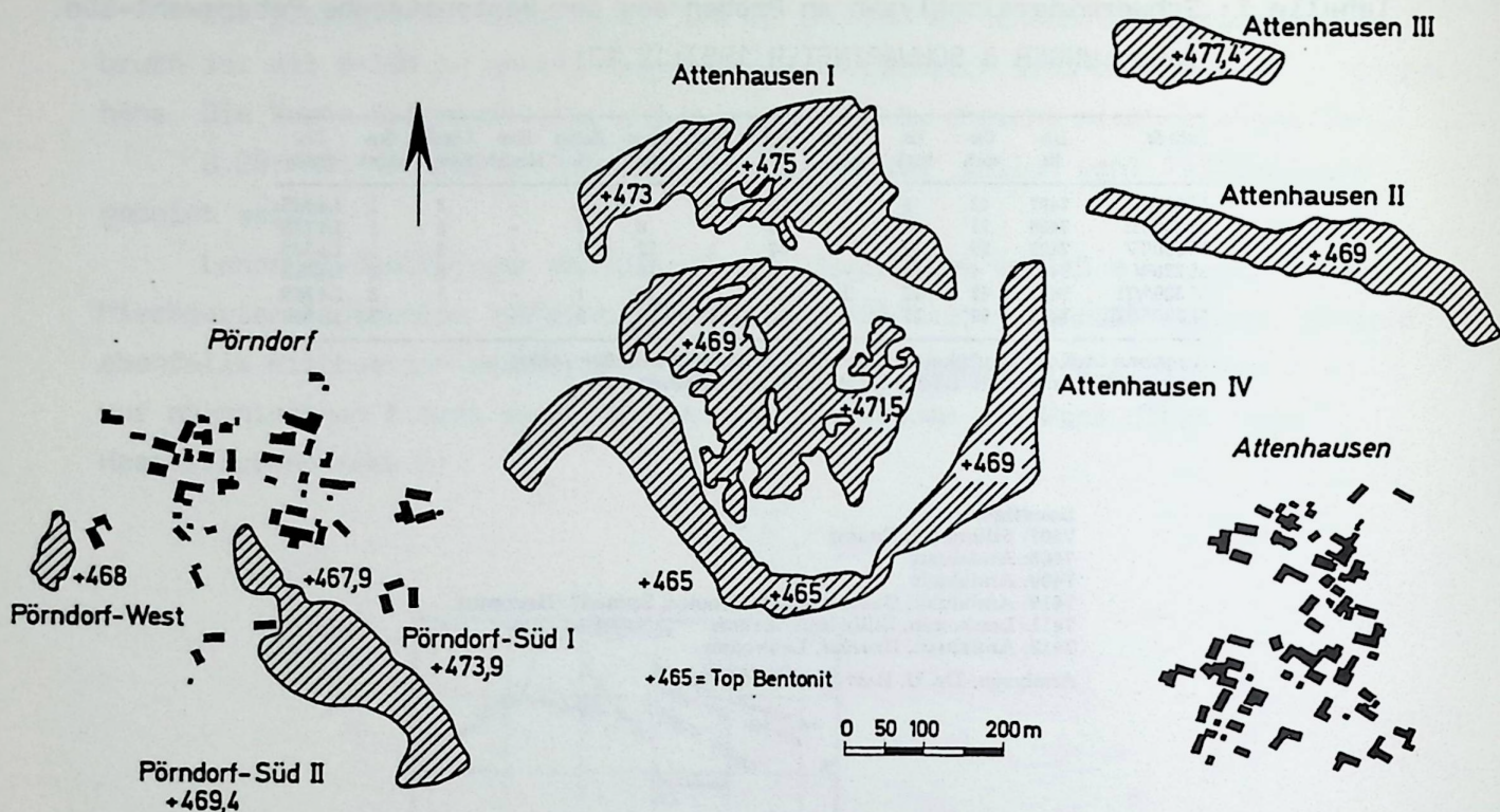
Abb.3. Lagerungsform (Altwässer, Seen, Tümpel) und Höhenlage (Basis) von Bentonitlagen zwischen Pörndorf und Attenhausen (nach alten Gruben- und Tagebau-Plänen der Südchemie A.G.). Die Höhendifferenz, z.T. innerhalb einer Bentonitlage, beträgt 2,0-6,0 m bis 8,4 m, also eine Höhen-Schwankungsbreite wie sie in jedem flachen Relief selbstverständlich ist.
