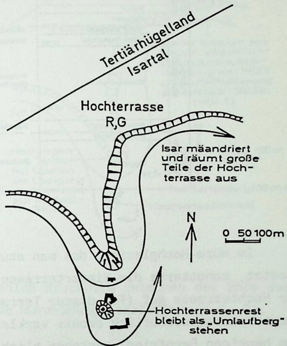
Abb.7. Die geologische Entwicklung um Schloß Bruckberg zwischen dem Ende des Mittelpleistozäns und dem Ende des Würm-Frühglazials (Phasen A,B).
