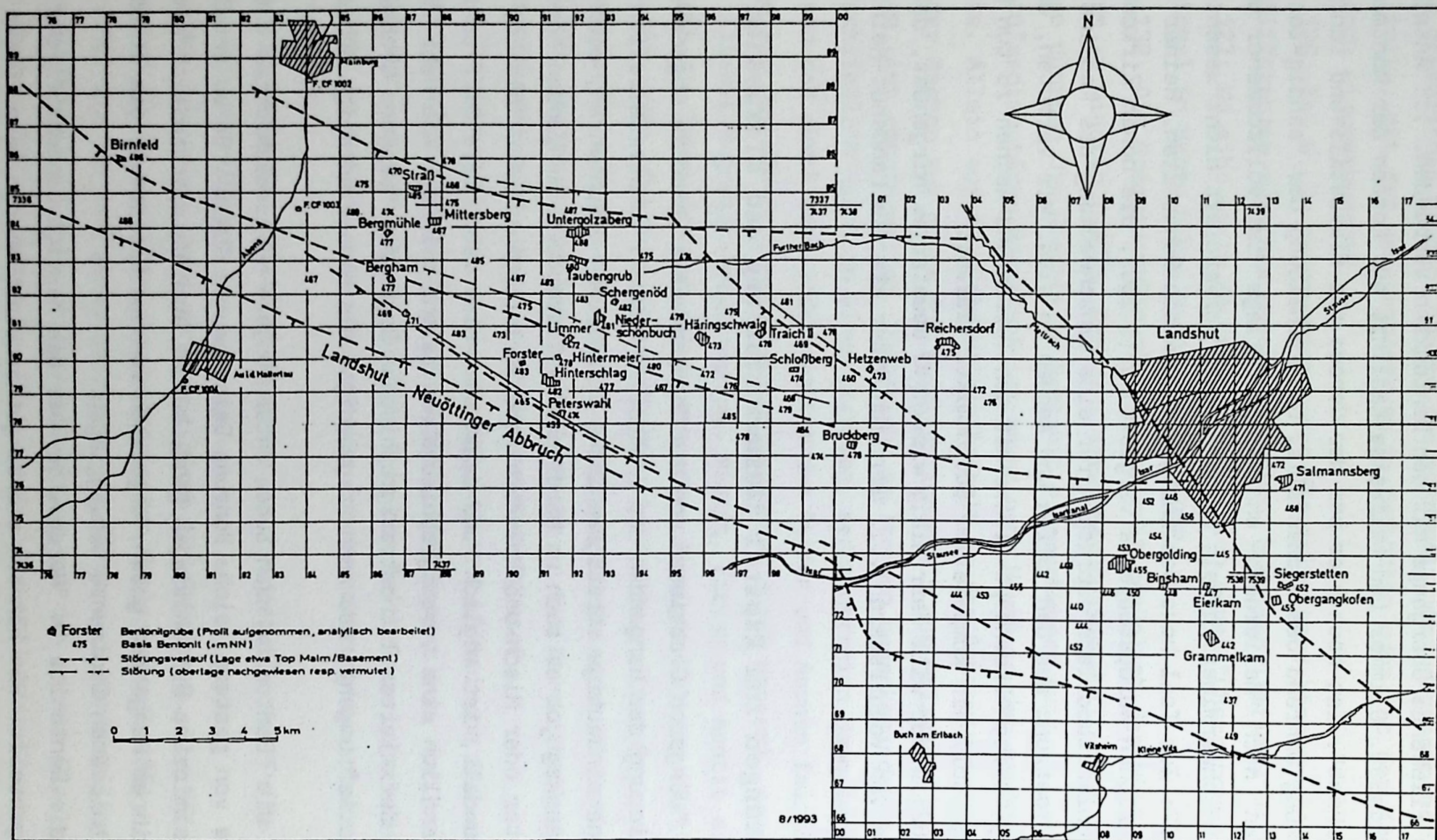
Abb.10. Tektonische Übersicht des Raumes Landshut-Mainburg mit Bentonitgruben.
