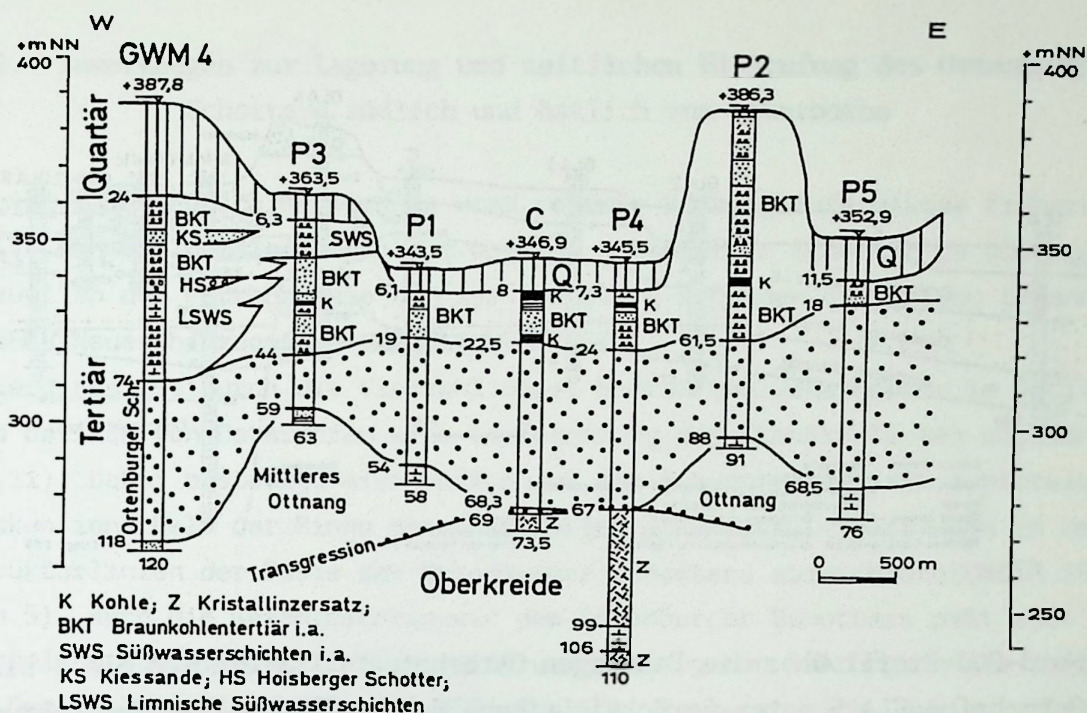
Abb.7. West-Ost-Profil über die Bohrungen Osterhofen Süd GWM 4 bis Osterhofen Süd P5 zur Verdeutlichung der Lagerung des Ortenburger Schotters und seines Liegenden und Hangenden (Legende und Lage der Bohrungen siehe Abb.3).
