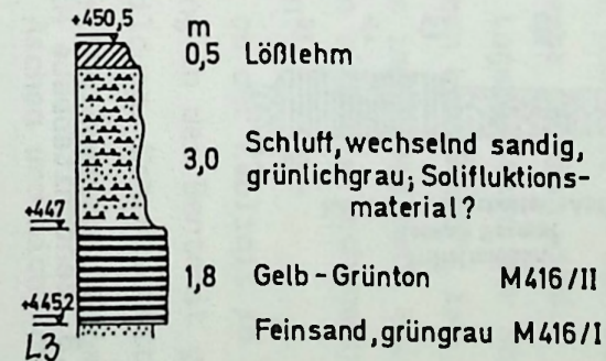
Abb.7. Bentonitabbau Bergmühle, Bergham, Schloßberg und Eierkam-Nord. Zur Lagerung des Plattentones und die Sedimente im Hangenden des Bentonits. Aufnahmen: H.J.Unger
