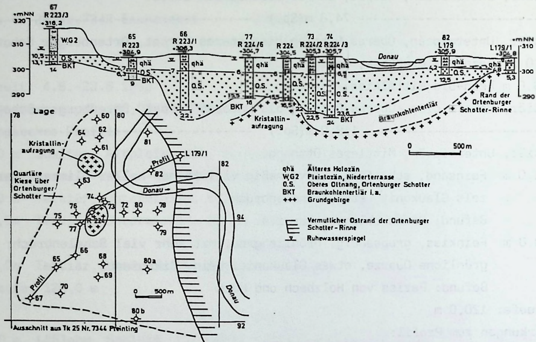
Abb.6. Lage und Profil von Bohrungen der Rhein-Main-Donau A.G.mit direkter Auflagerung quartärer Terrassenkiese auf Ortenburger Schotter nördlich von Pleinting
