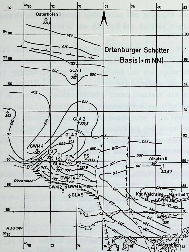
Abb.10. Strukturlinien Basis Ortenburger Schotter südlich von Osterhofen
