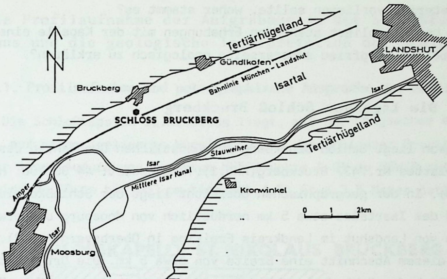
Abb.2. Geographische Lage von Schloß Bruckberg im Isartal
