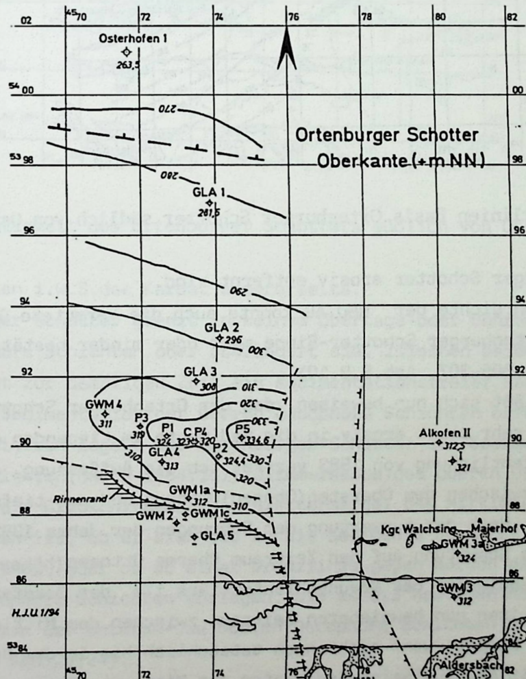
Abb.9. Strukturlinien Oberkante Ortenburger Schotter südlich von Osterhofen nach neueren Bohraufschlüssen
