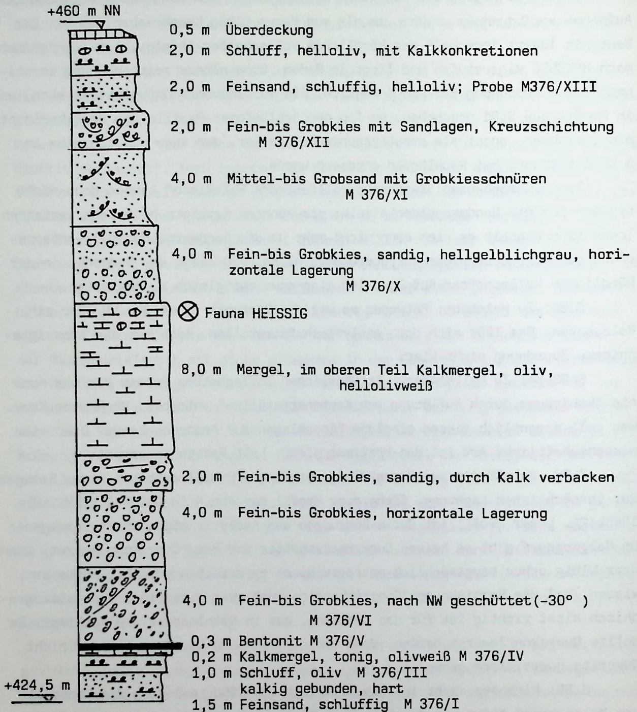
Abb.9. Kurzprofil des Aufschlusses Kiesgrube Artlkofen. Aufnahme: H.J.Unger
