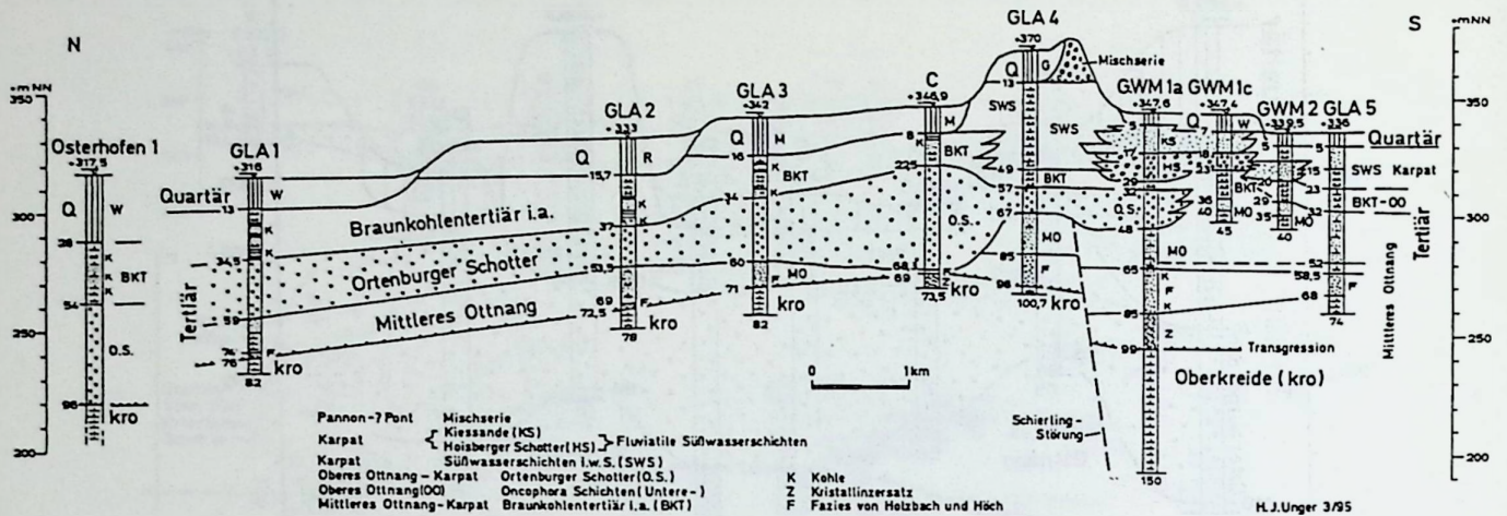
Abb. 8. Nord-Süd-Profil über die Bohrungen Osterhofen 1, Osterhofen GLA 1 bis Osterhofen GLA 5 unter Berücksichtigung der Bohrergebnisse der Bohrungen Osterhofen Süd C, GWM 1a, GWM 1c und GWM 2 ( Q-W,R,M,G = Quartär-Niederterrasse, Hochterrasse, Mindelzeitliche Terrasse und Günzzeitliche Terrasse)(Lage des Profils siehe Abb.3).
