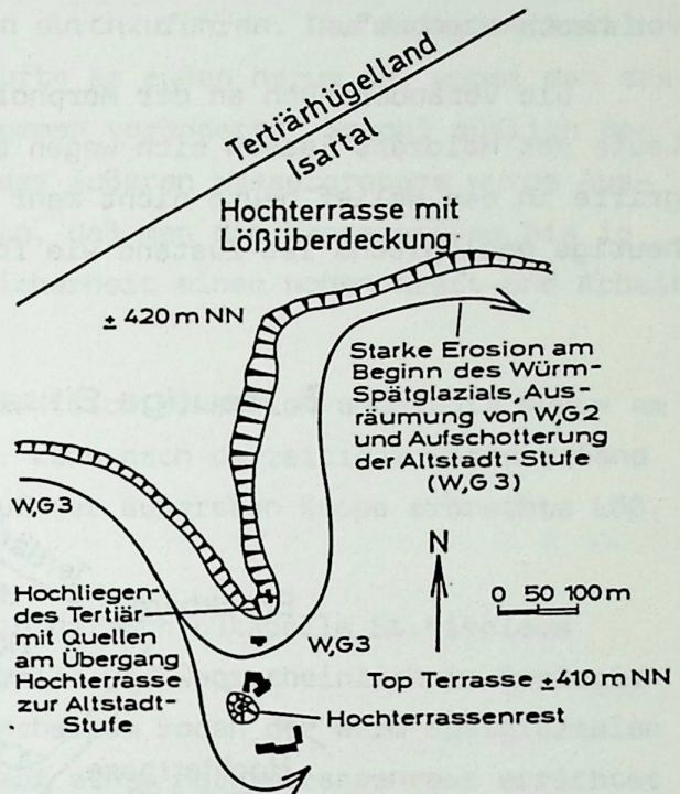
Abb.8. Die geologische Entwicklung um Schloß Bruckberg zwischen dem Ende des Würm-Hochglazials und dem Ende des Würm-Spätglazials (Phasen C, D).
