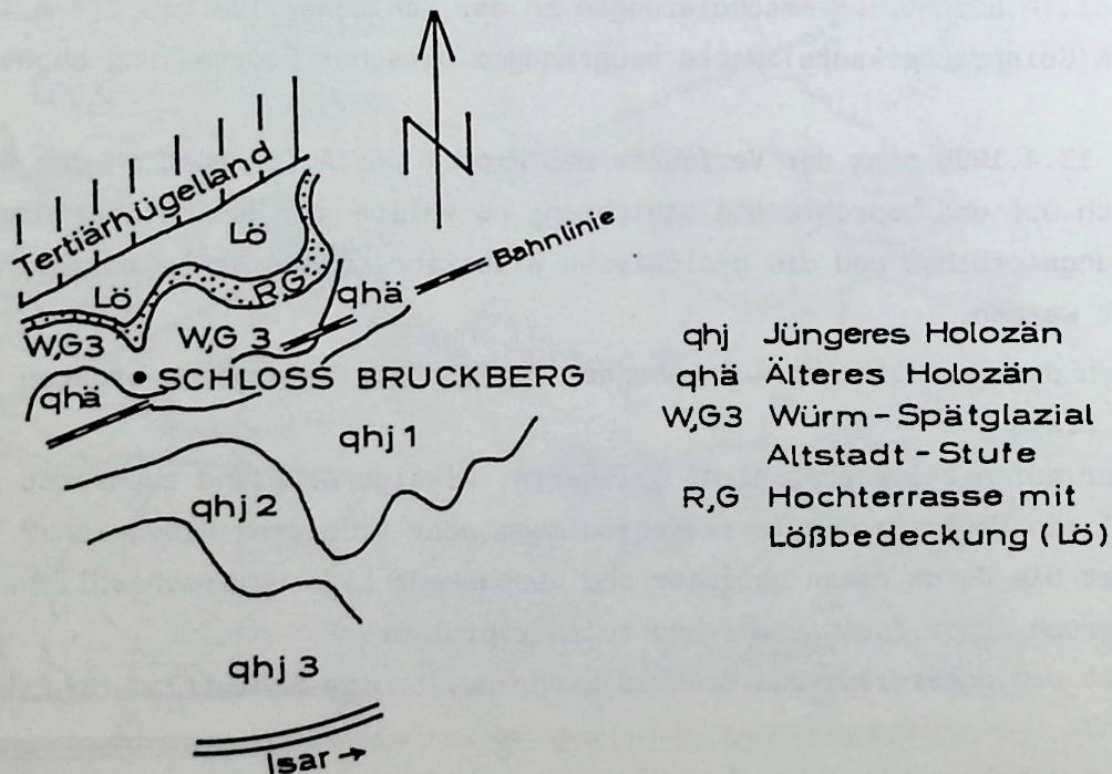
Abb.3. Geologische Übersicht der näheren Umgebung von Schloß Bruckberg
