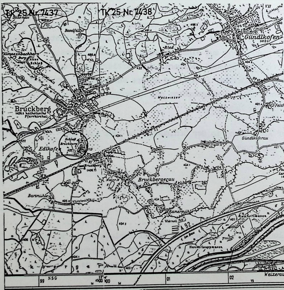
Abb.1. Topographische Lage von Schloß Bruckberg im Südostquadranten des Gradabteilungsblattes Nr.7437 Bruckberg
