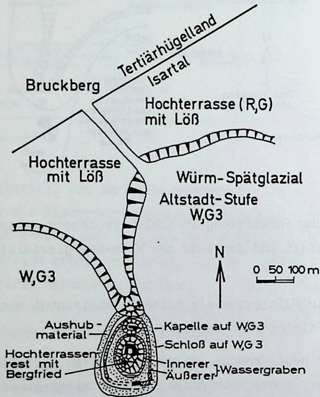
Abb.9. Die heutige geologische Situation um Schloß Bruckberg
