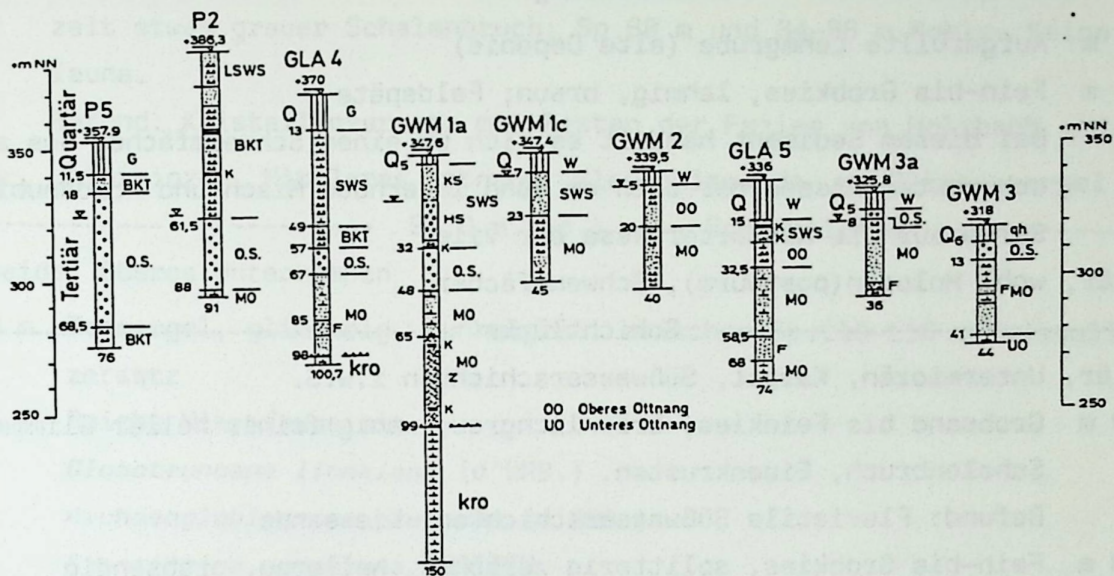
Abb.4. Geologische Kurzprofile der Bohrungen Osterhofen Süd P5 bis Osterhofen Süd GWM 3 (Legende und Lageplan der Bohrungen siehe Abb.3.).
