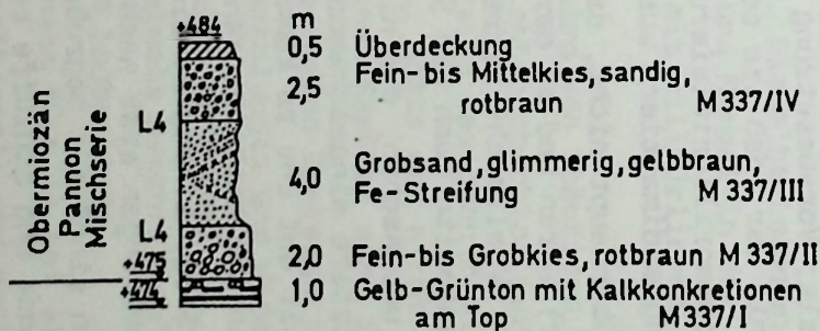
Abb.7. Bentonitabbau Bergmühle, Bergham, Schloßberg und Eierkam-Nord. Zur Lagerung des Plattentones und die Sedimente im Hangenden des Bentonits. Aufnahmen: H.J.Unger
