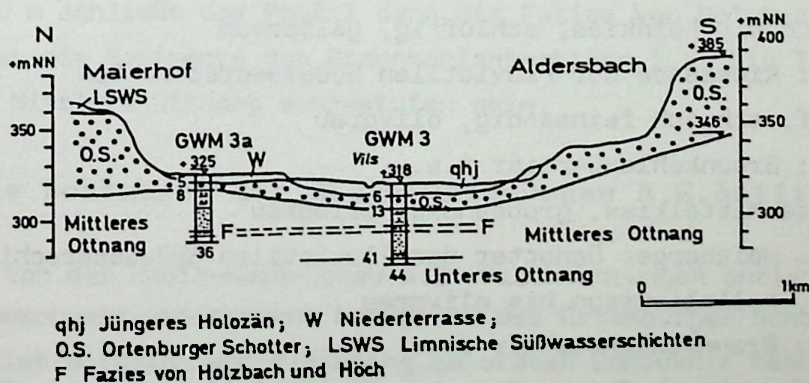
Abb.5. Nord-Süd-Profil über das Vilstal nördlich von Aldersbach mit den Bohrungen Osterhofen Süd GWM 3a und GWM 3.
