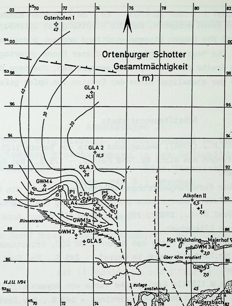
Abb.11. Mächtigkeit des Ortenburger Schotter südlich von Osterhofen
