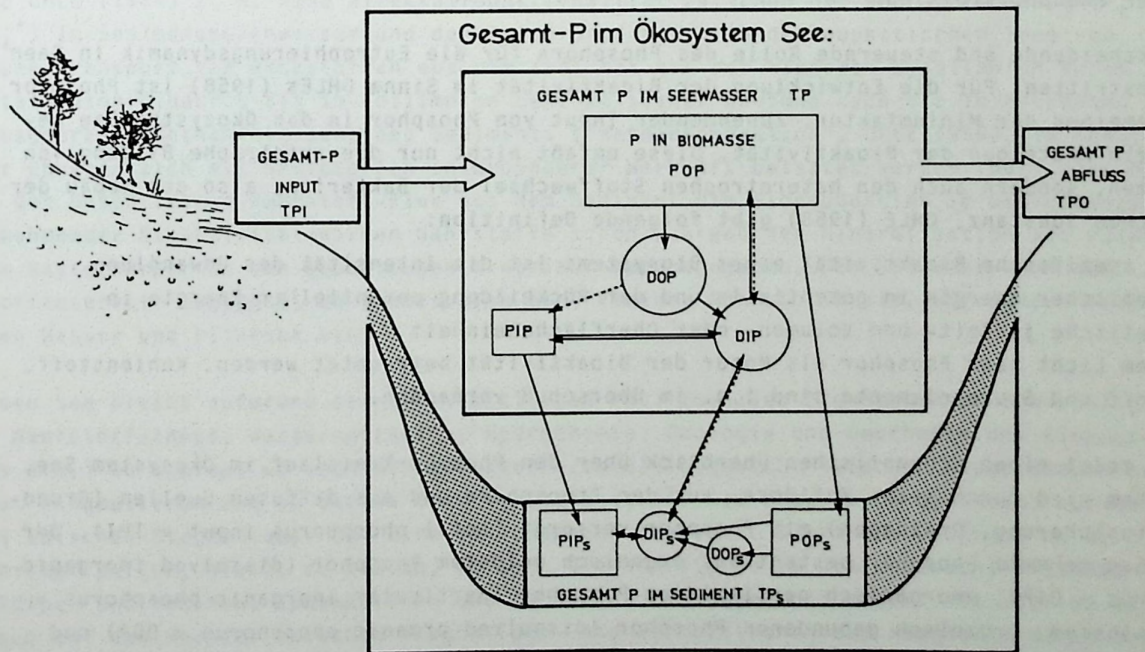
Abb. 38 P-Kreislauf (schematisch) im ÖKOSYSTEM SEE
