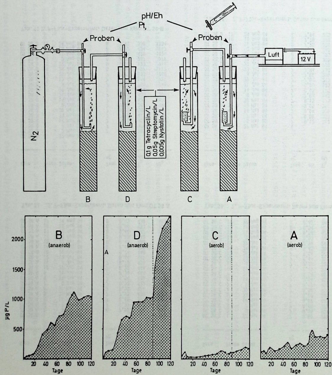
Abb. 42 Versuchsaufbau und Verlauf des 2. P-Flux - Experiments
