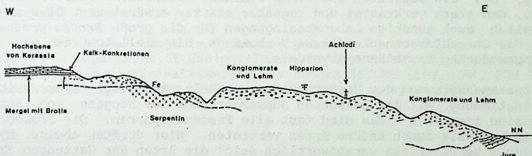
Abb. 1: Schnitt im Neogen vom Plateau von Kerassia bis zum Meeresufer bei Achladi (N-Evia). Nach GUERNET (1971).
