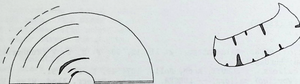
Abb. 2: Schematische Darstellung der Mündungslamellen bei Strobilops labyrinthica von Kerassia.
