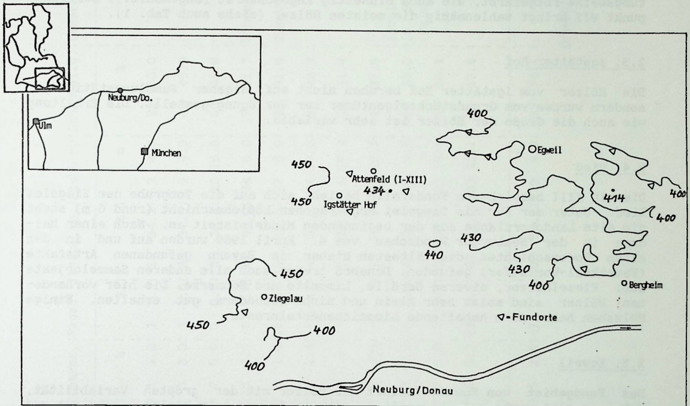
Abb. 1: Geographische Lage des Fundgebietes
