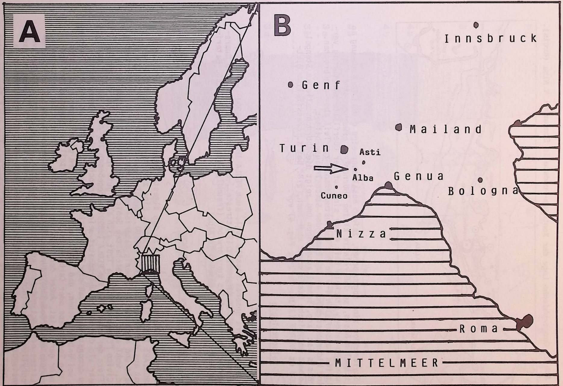
Abb.1: Europakarte (A) mit Angabe der Fundregion (senkrecht schraffiertes Quadrat) und Ausschnitt von Oberitalien (B) mit der Provinz Turin (Torino) und der Fundstelle bei Alba (Pfeil).
