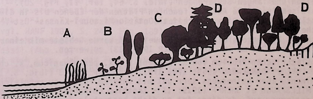
Abb.6: Versuch einer Rekonstruktion der fossilen Faziesverhältnisse von Scaparoni im Messin mit Offenem Wasser, Strandzone und trockenem Hochland mit einem mesophytischen Wald.
