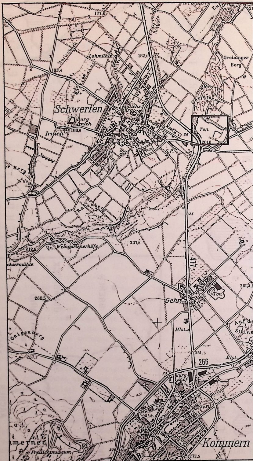
Abb.3: Lage der Tongrube östlich Schwerfen bei Zülpich.
