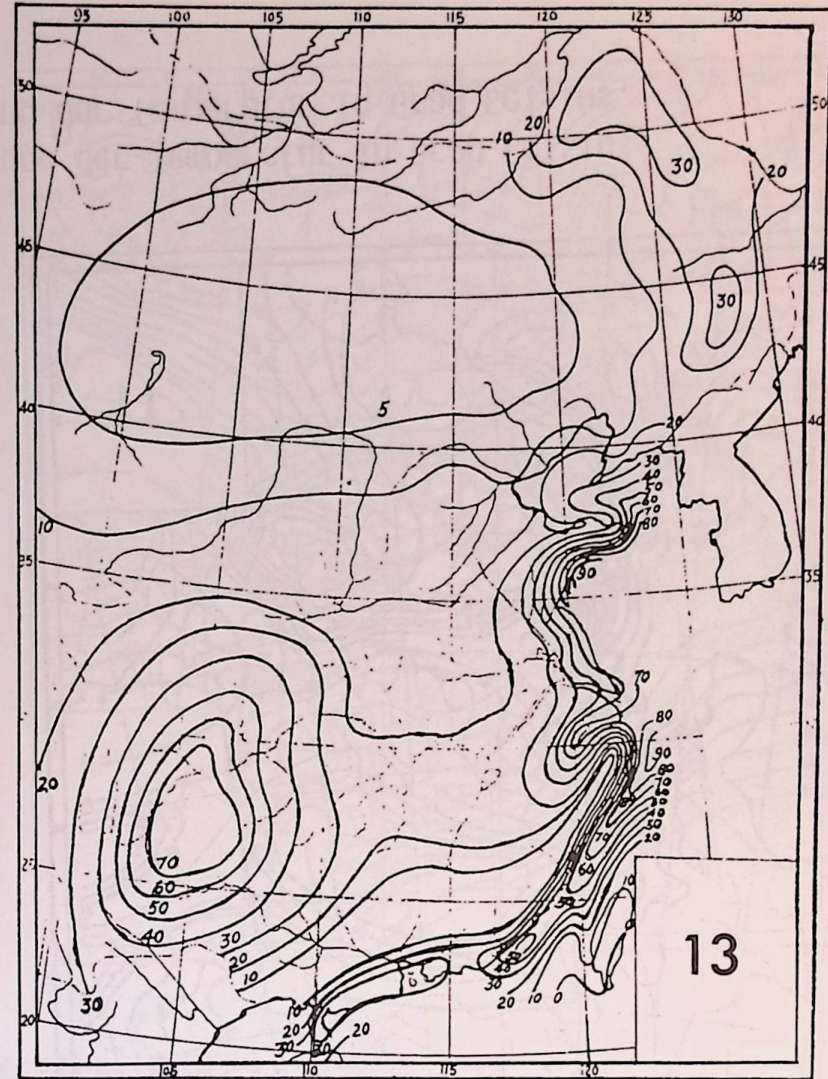
Abb.12: Mittlere jährliche relative Feuchtigkeit in Prozent. Abb.13: Mittlere jährliche Anzahl nebliger Tage.
