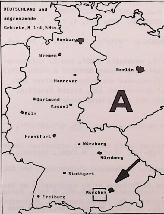
Abb.1: Geograpische Lage der Fundstelle Kiesgrube Bauer in Hilpoldsberg bei Schwabmünchen; A=Lage in Süddeutschland;B= Lage auf der Molassekarte-GREGOR 1982;C=auf der TK 7728 (M 1:50 000).
