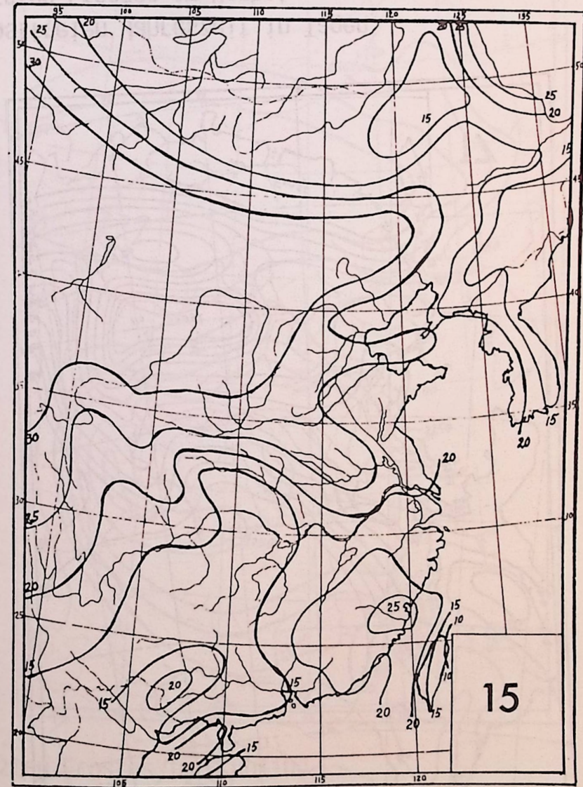
Abb.15: Mittlere jährliche Reichweite der Niederschlagsvariation in mm.
