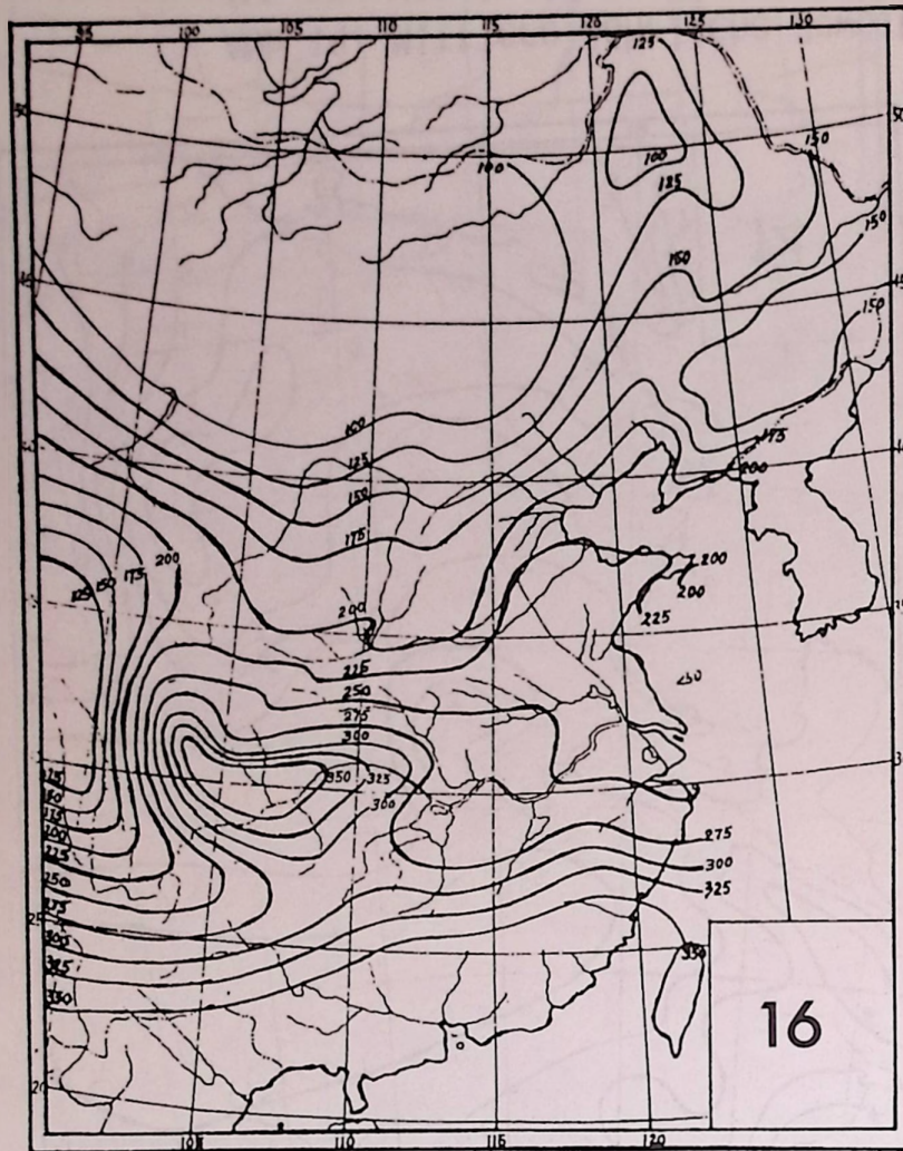
Abb.16: Mittlere Länge der frostfreien Jahreszeit in Tagen. Abb.17: Mittleres Datum des ersten Frostes im Herbst.
