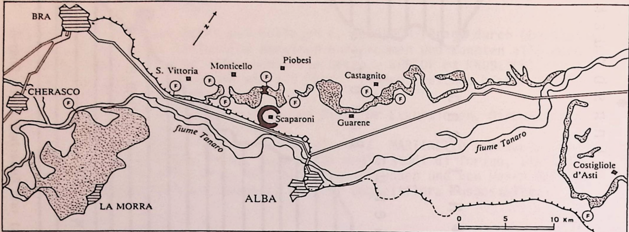
Abb.2: Geographische Lage der Xanthium-Fundstelle Scaparoni N Alba (Kreis).
