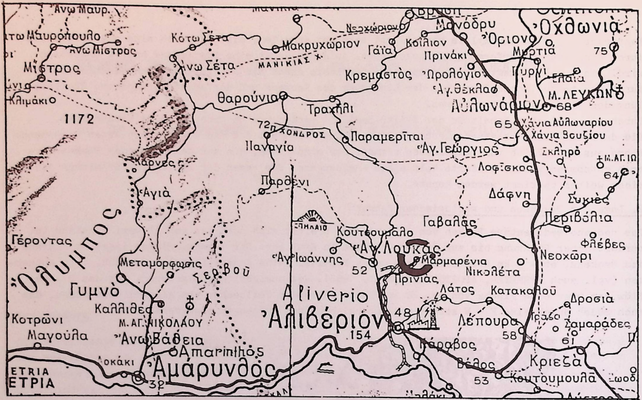
• Abb.1 B: Lage des Untersuchungsgebietes nördlich Aliveri (M 1:200 000).
