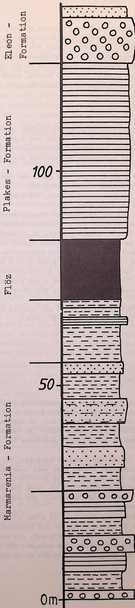
Abb.2: Schematisches Schichtenprofil im Tagebau Plakes (Aliveri).
